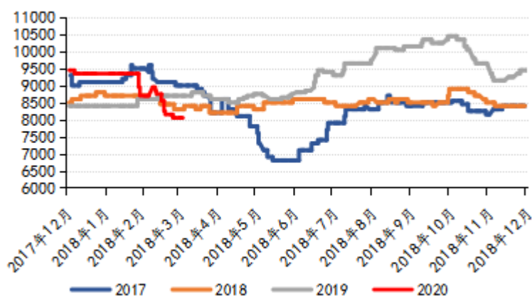
Mysteel-304废不锈钢价格：温州（元/吨）
