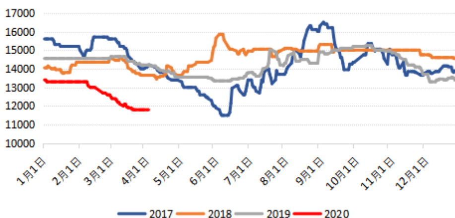
Mysteel-北海诚德：佛山市场价格：不锈热卷： 304/NO.1：5*1500*C（日）
