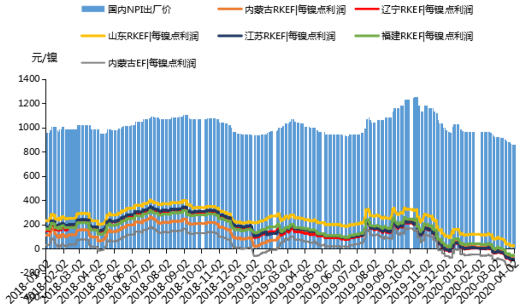
Mysteel-国内镍铁即期利润
