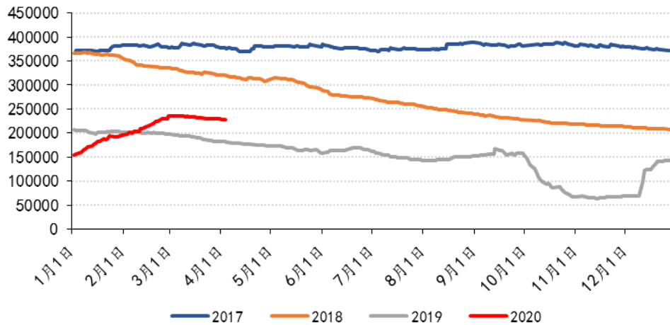
LME库存合计：镍（吨）
