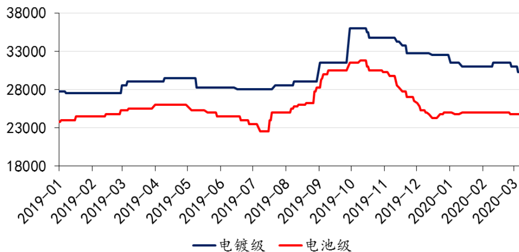
Mysteel-国内硫酸镍价格统计 (元/吨)
