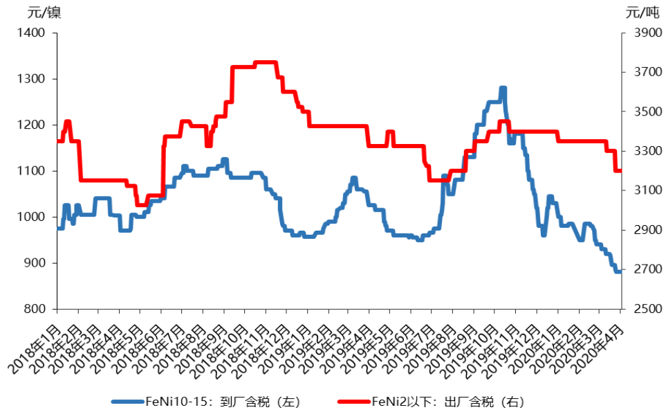
Mysteel-镍铁价格
