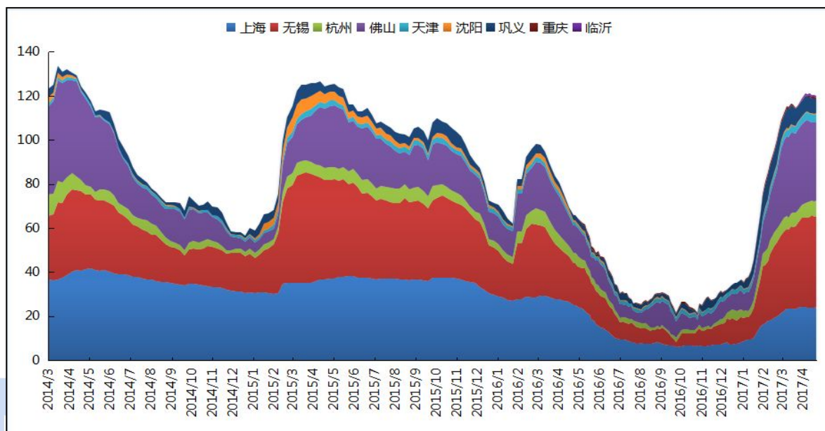
图三、 国内主流市场电解铝库存统计图(万吨)
