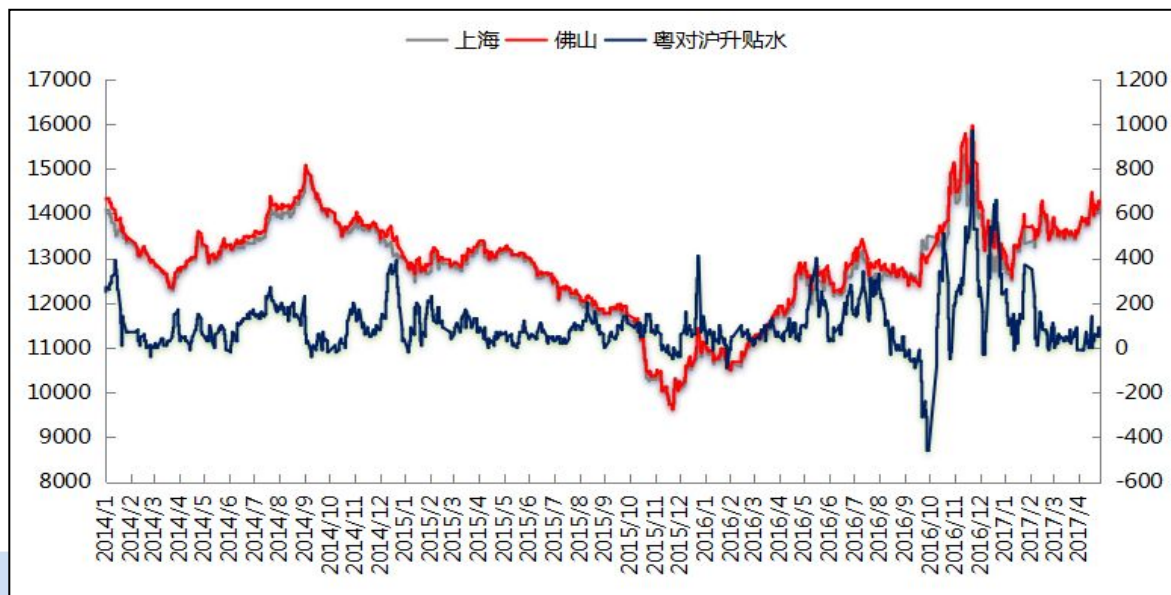
图二、 沪粤两地现货铝锭价格走势对比图
