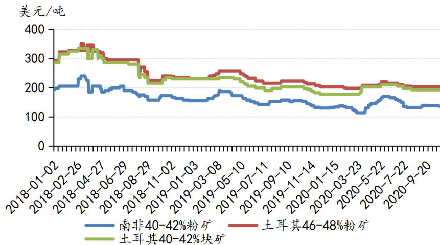
Mysteel-铬精矿外盘价格走势
