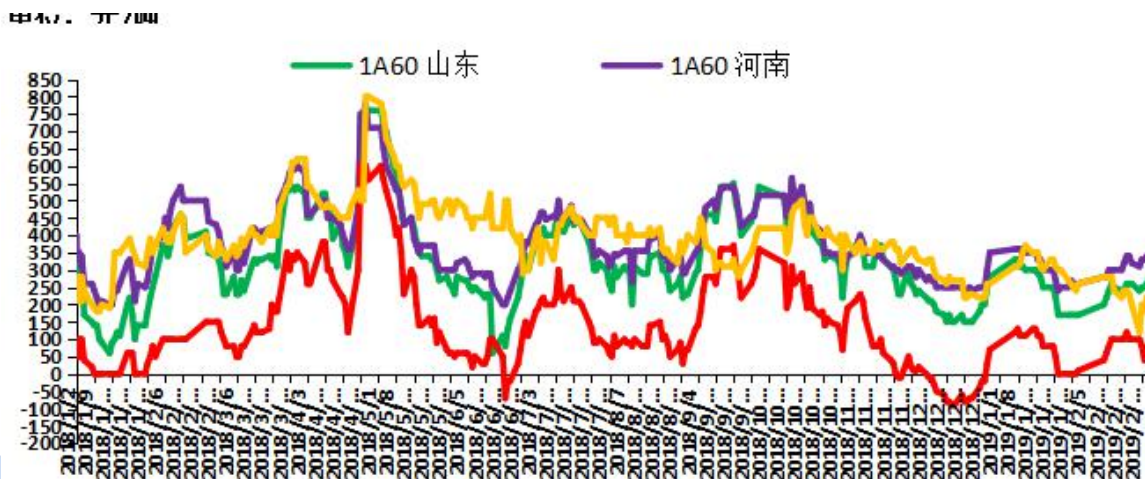
图 1. 2016-2018 年全国主流地区 1A60 电工圆铝杆价格走势图
